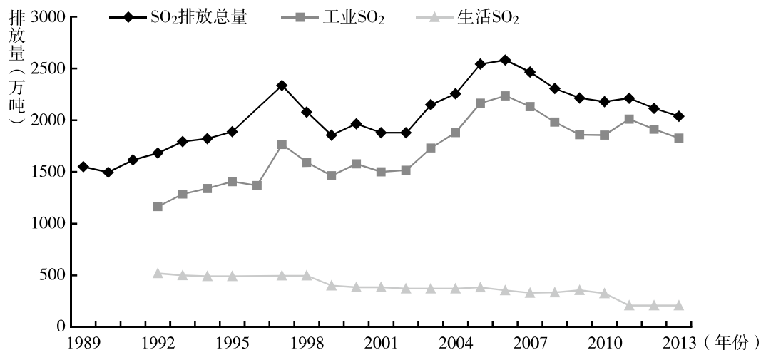
图3 中国SO 2 排放量的变化趋势
