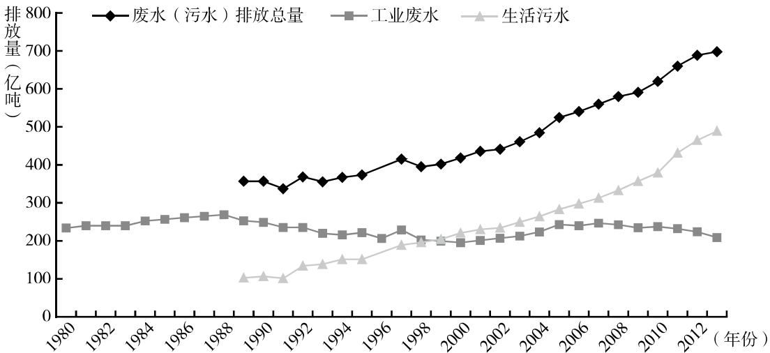
图 1 中国废水（污水）排放量的变化趋势
