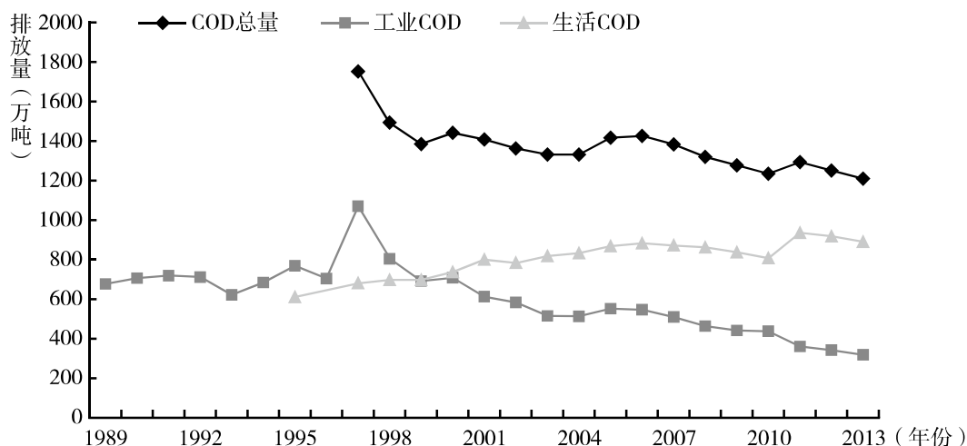
图2 中国COD排放量的变化趋势
